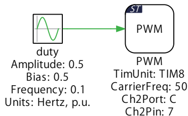
図5: PWMブロックを使用してG474REのLEDを調光する回路図
