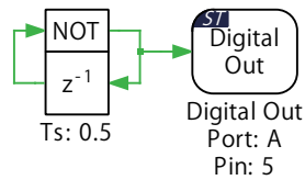
図1: G474REのLEDを点滅させる回路図
