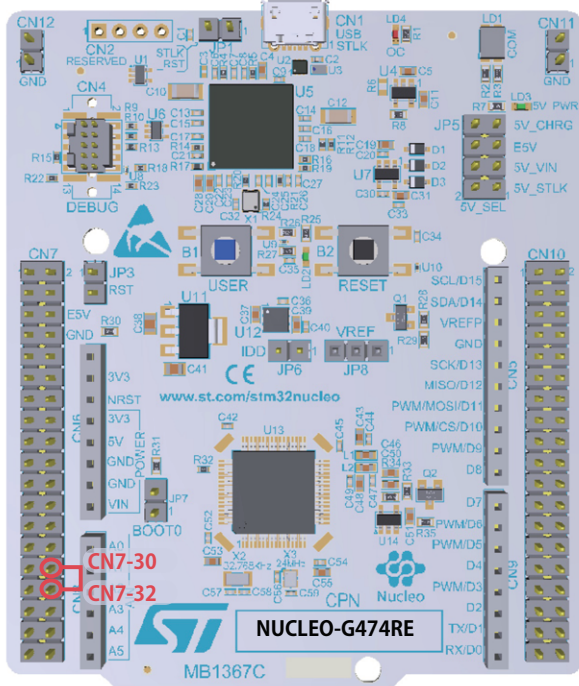
図10: ジャンパ線を使用してピンCN7-32をCN7-30に接続
