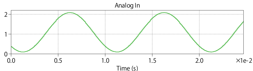
図11: Nucleo-G474REでキャプチャしたリアルタイムADC信号
