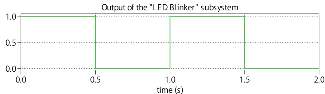
図3: PLECS上で"LED Blinky"サブシステムをオフラインで実行した結果
