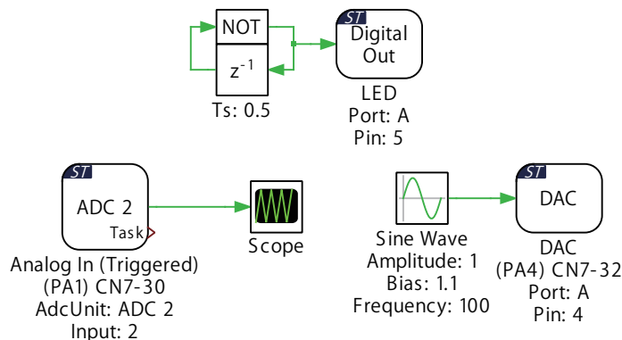
図8: Analog Loopbackサブシステムの回路図
