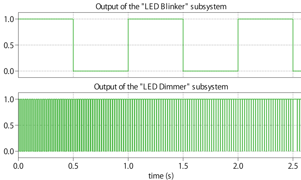
図7: PLECSにおける"LED Dimmer"サブシステムのオフラインテスト結果
