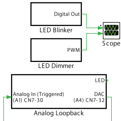
図9: トップレベルの回路図
