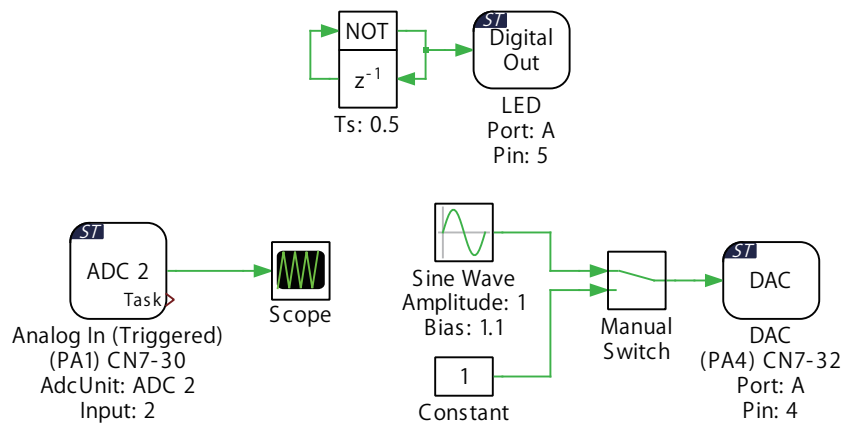
図12: 編集したAnalog Loopbackサブシステムの回路図
