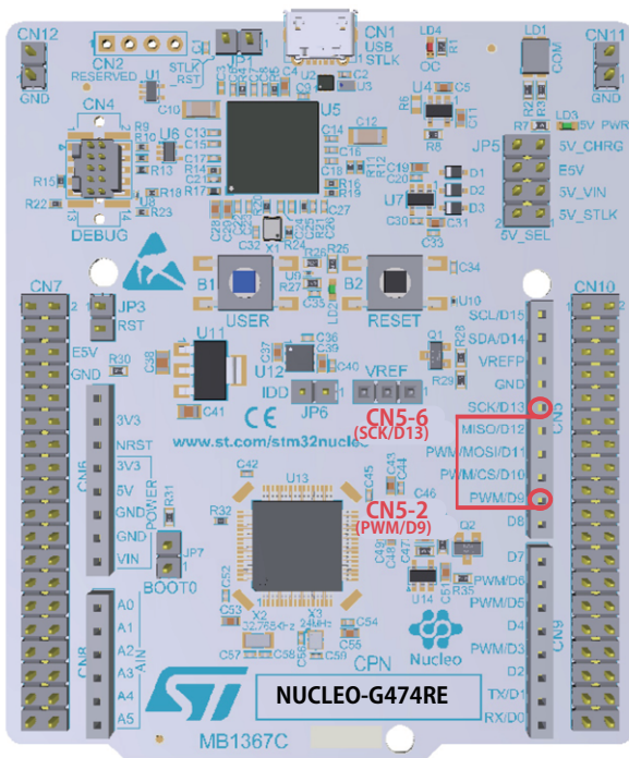
図4: ジャンパ線を使用してPWM出力(CN5-2)をLED "LD2"(CN5-6)に接続
