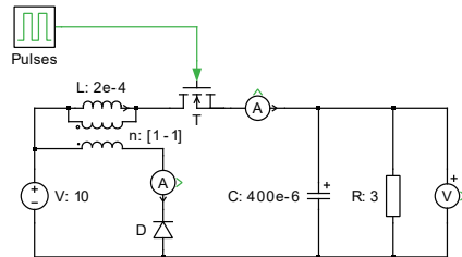
図1: 2つの巻線を備えたWJコンバータ
