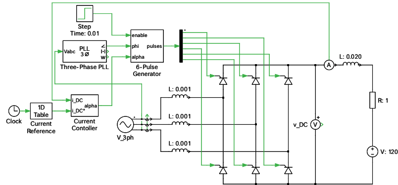
図1: フィードバック制御の三相グリッド接続サイリスタ(SCR)整流器
