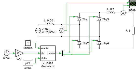
図1: RL負荷を備えた2パルス単相サイリスタコンバータ
