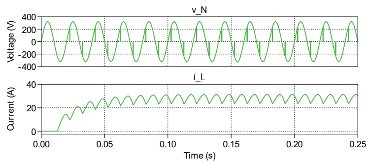
図2: 入力電圧前のサイリスタコンバータと負荷電流のシミュレーション結果
