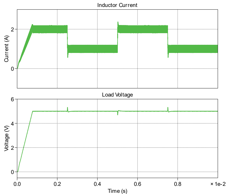
図3: 負荷ステップ下の閉ループにおける同期降圧コンバータのシミュレーション結果
