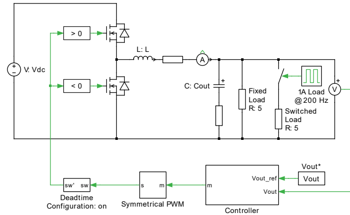
図1: 同期降圧コンバータ
