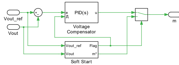
図2: 制御システムの最上位レベルの回路図
