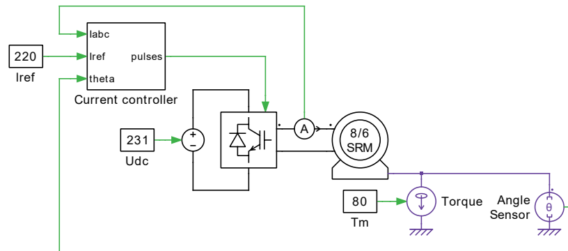
図1: SRモータ(8/6)回路
