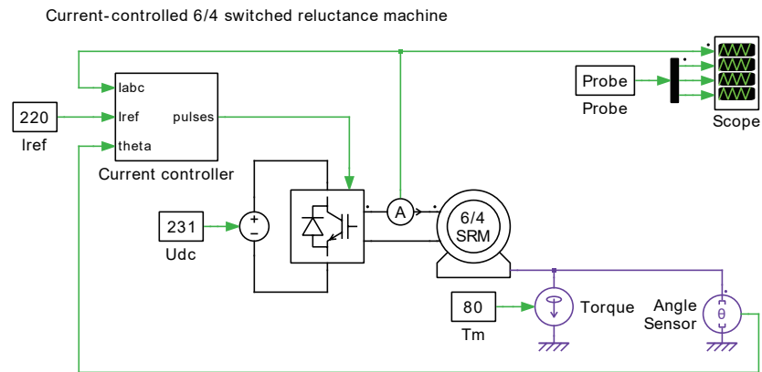
図1: SRモータ(6/4)回路
