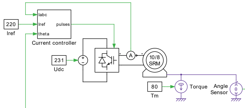
図1: SRモータ(10/8)回路
