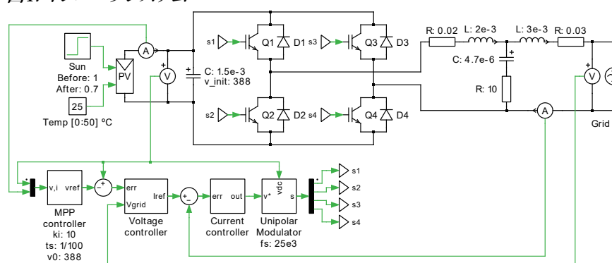
図1: インバータシステム
