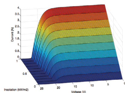
図2: 25°CにおけるBP365 PVモジュールモデルの代表的な出力電流特性
