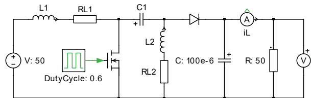
図1: SEPICの回路図
