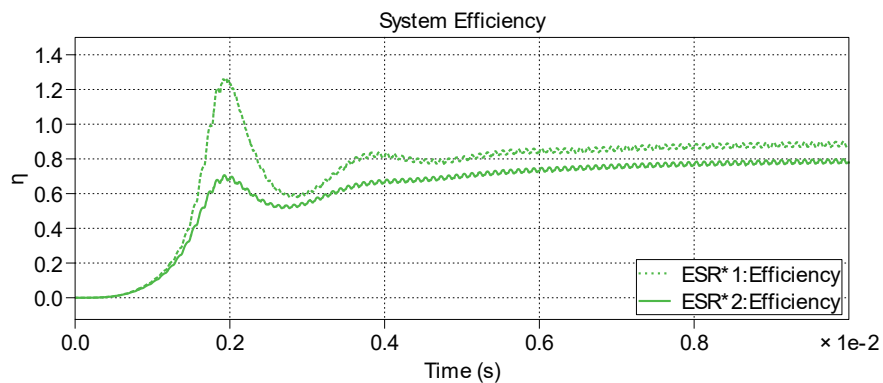
図2: 異なるESR値におけるシステム効率の結果
