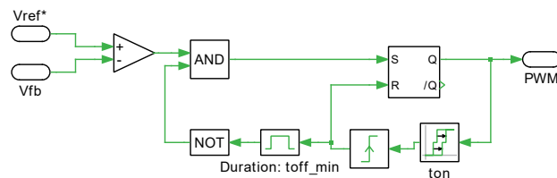
図2: コントローラの回路図
