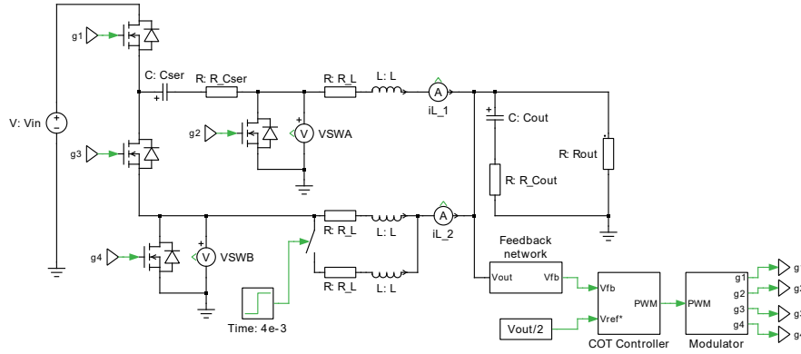
図1: COT制御を備えた2相直列キャパシタ降圧コンバータ回路
