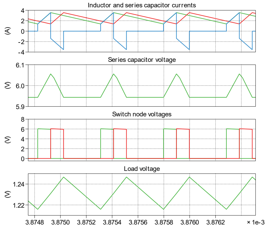
図3: 定常動作におけるシミュレーション結果
