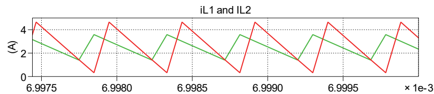
図4: 平均インダクタ電流
