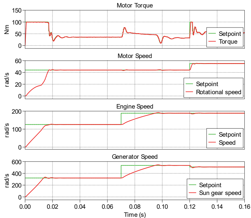
図4: PLESCプローブのMechanicalの波形
