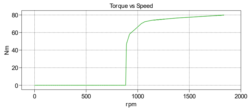
図6: トルク速度曲線
