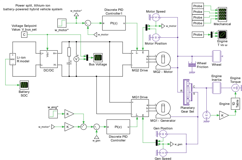
図1: 全体的なシステムモデル
