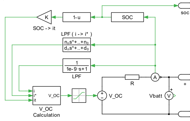
図2: Li-ion R modelサブシステム
