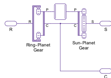
図3: 遊星ギアサブシステム
