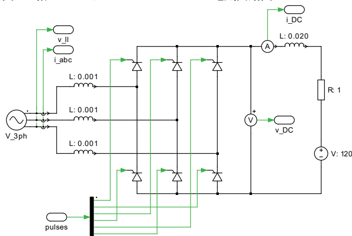
図1: 3相6パルスサイリスタコンバータの電気回路図
