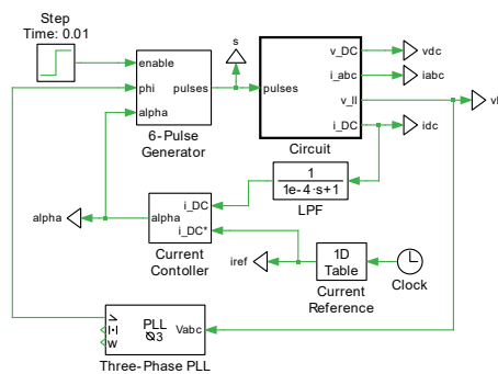
図3: 生成されたコードを使用してモデル化された"Circuit"サブシステムの制御回路図
