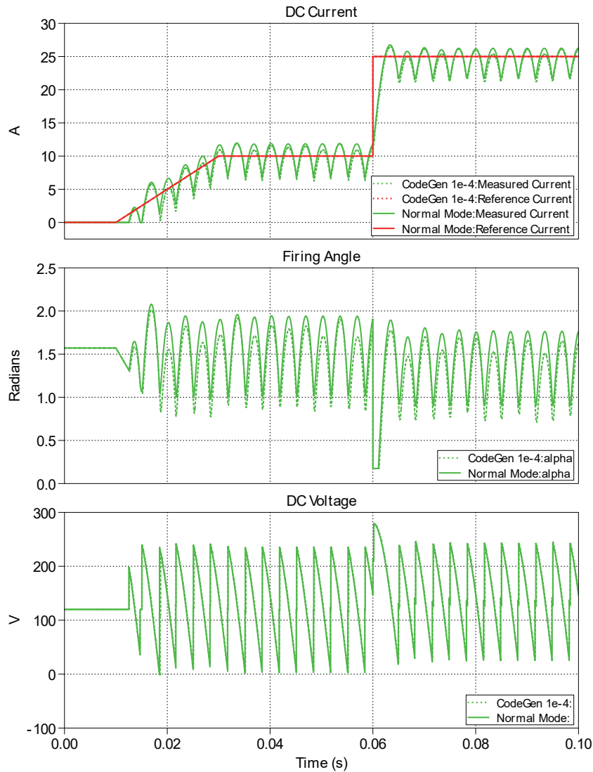
図4: "Normal Mode"と"CodeGen 1e-4"の比較結果
