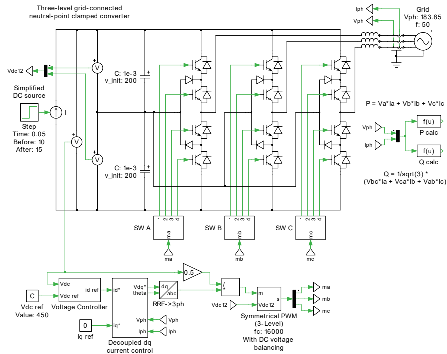
図1: NPCコンバータ
