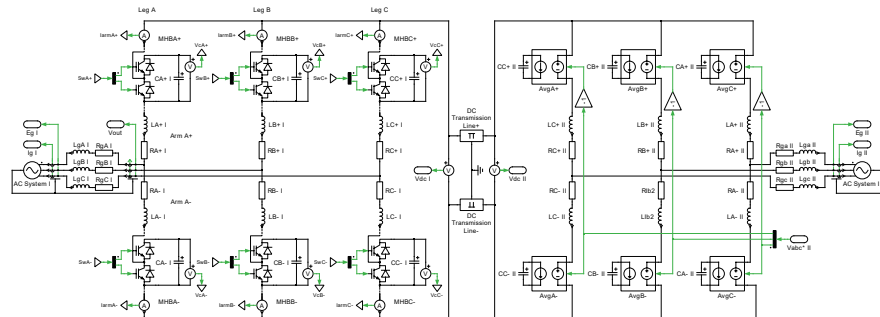
図1: MMC系統連系とDC送電線を備えたHVDCシステム
