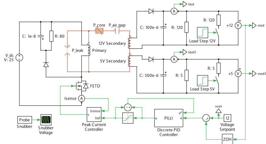
図1: 磁気回路を備えた3出力フライバックコンバータの回路図
