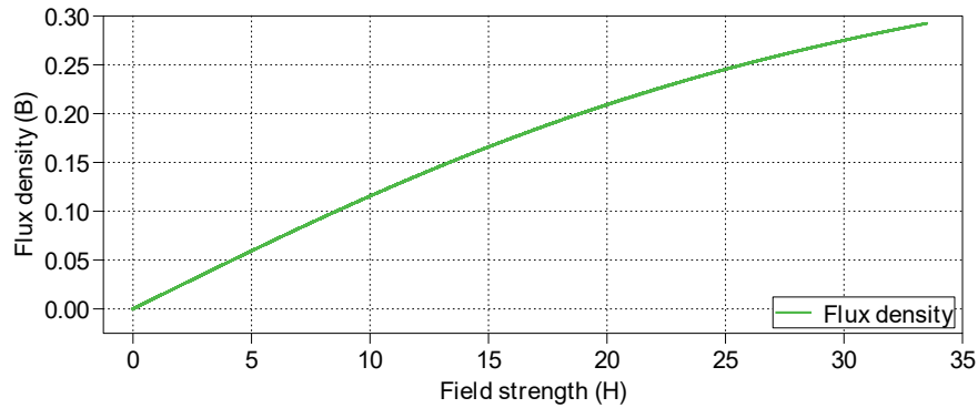
図2: 3C91材料で作られたFerroxcube 2616ポットコアの飽和曲線
