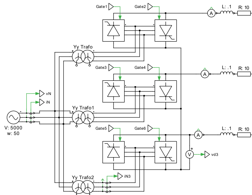
図1: サイクロコンバータ
