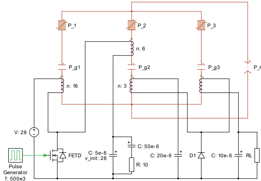
図1: 磁気回路を備えたCukコンバータ
