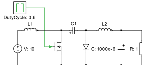
図1: Ćukコンバータ
