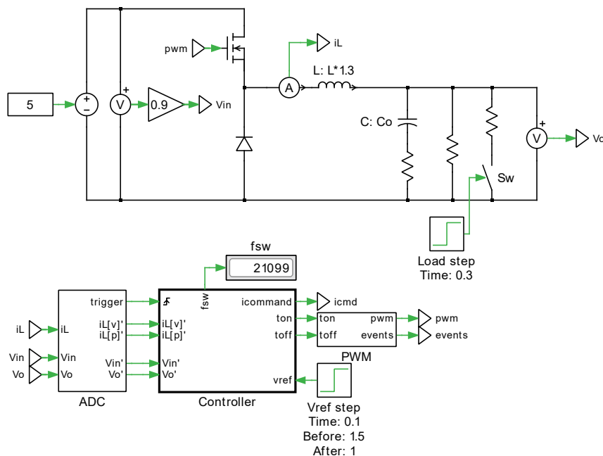
図1: モデルのトップレベルの回路図
