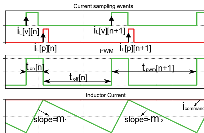
図3: BCMによる予測電流制御
