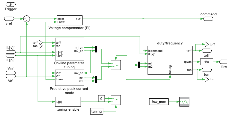
図2: BCMの降圧コンバータのコントローラ
